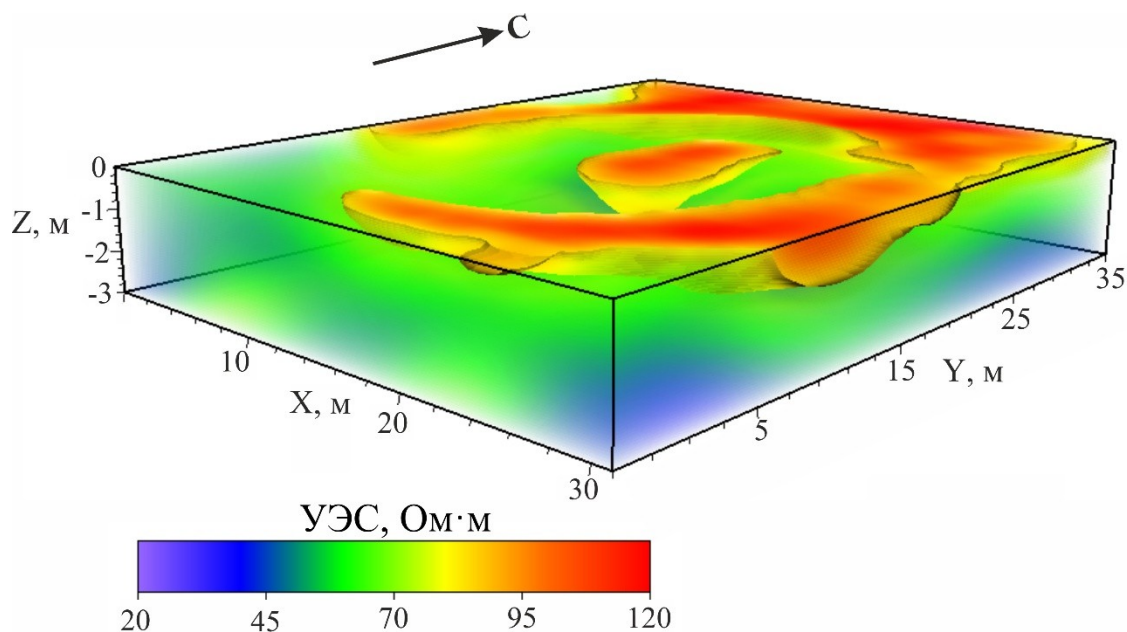
Рисунок 4. Трёхмерная геоэлектрическая модель кургана на могильнике Конево-10 по результатам 2D измерений.
