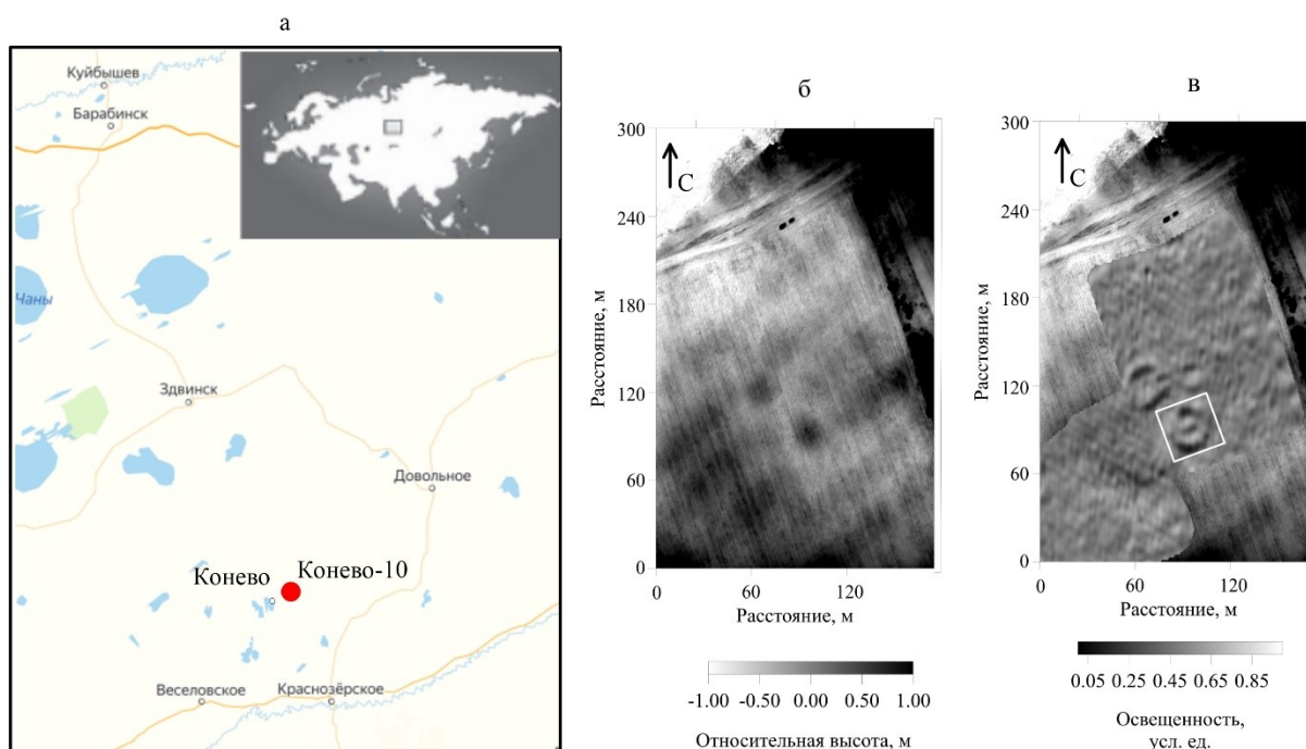
Рисунок 3. Карта района работ (а). Карта относительных высот археологического памятника (б) и теневая карта распределения реальной компоненты сигнала с горизонтальным и вертикальным углами искусственного освещения в 126^\circ и 29^\circ (в).
