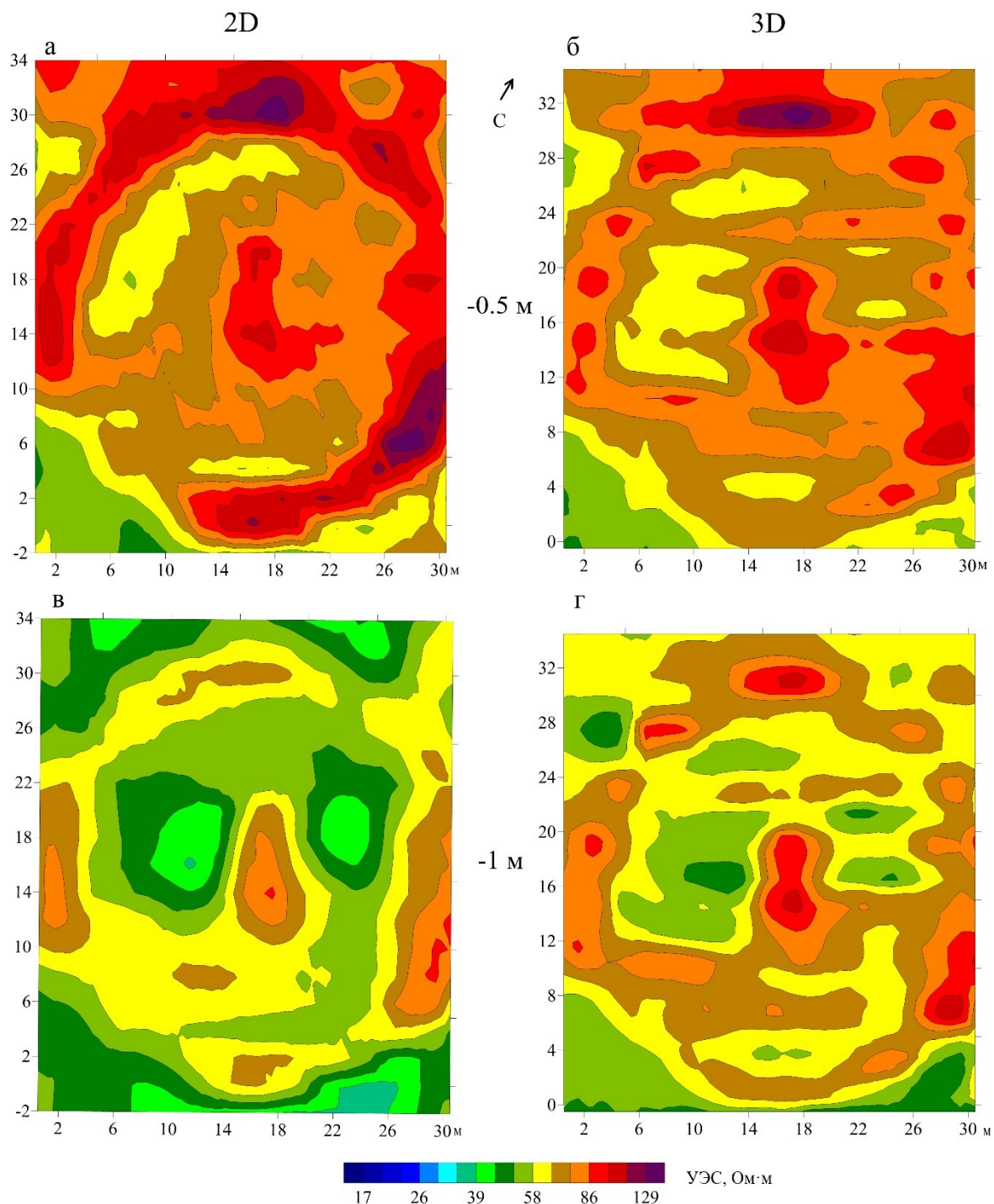
Рисунок 5. Срезы для массивов двумерных и трехмерных данных на двух глубинах: а – 2D данные на глубине 0.5м, б – 3D данные на глубине 0.5м, в - 2D данные на глубине 1м, г – 3D данные на глубине 1м.
