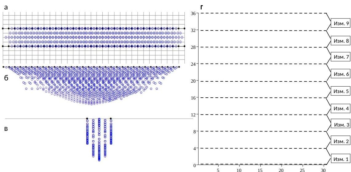
Рисунок 2. Система 3D измерений, синим – точки записи, черным – электроды. Слева общее облако точек записи, где, а – плоскость XY, б – плоскость XZ, в – плоскость ZY; г – схема трехмерных измерений (вид сверху), пунктирные линии – схематично показаны электроразведочные косы.
